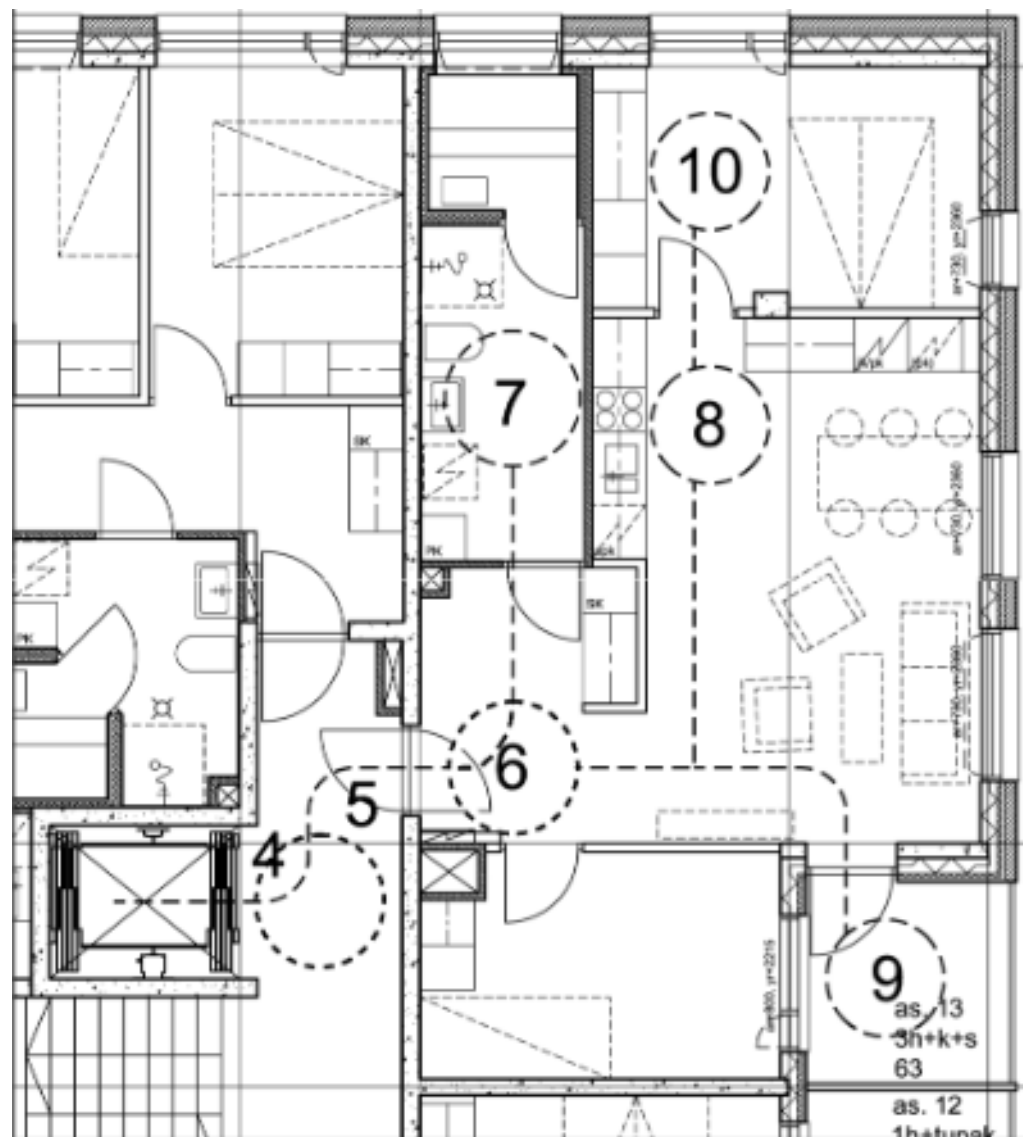
Pohjapiirustusote 2.krs // 1:100
